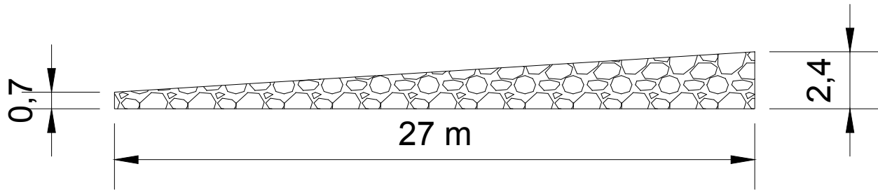
ALÇAT DEL MUR
